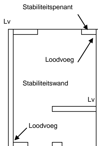
Plattegrond rijtjeswoning
