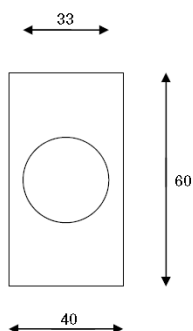
BOVENAANZICHT
