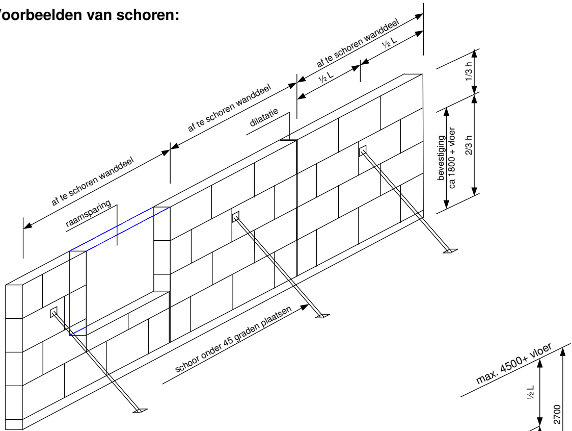
Figuur 4. Voorbeeld 1 Wand met dilatatie en raamopening
