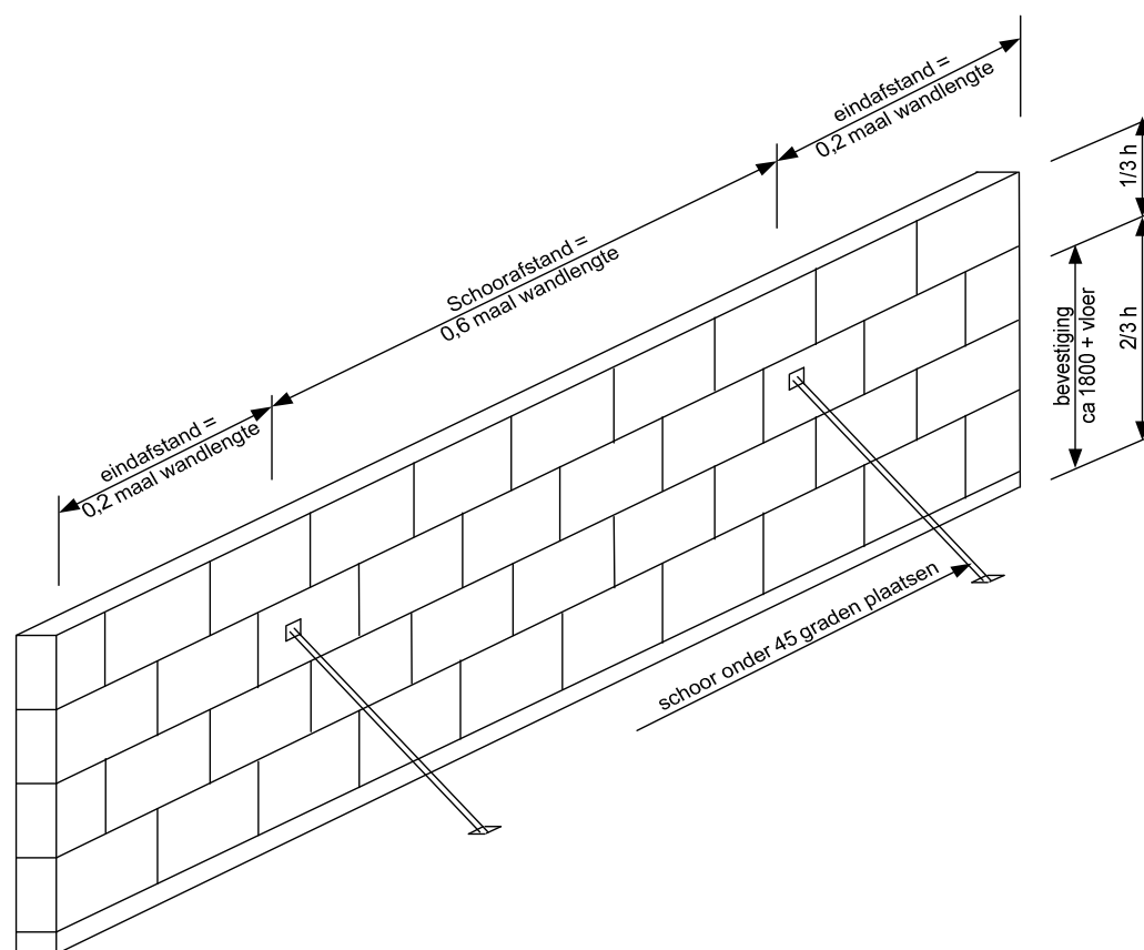
Figuur 1. Schoren van rechthoekige wanden met meerdere schoren.
